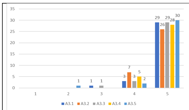
SDSAI (N=33)
