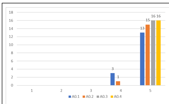
SDSAI (N=16)
