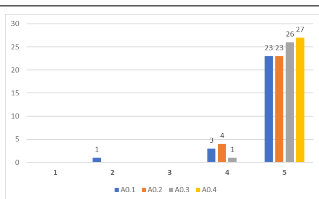
SDSSU (N=27)
