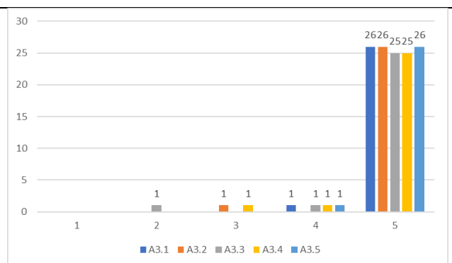
SDSSU (N=27)
